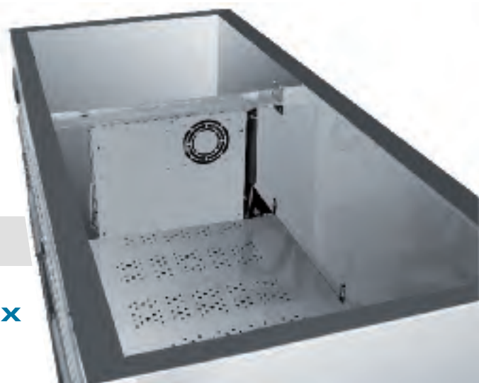
Esempio di installazione di evaporatore ventilato fissato trasversalmente. Example of installation of ventilated evaporator fixed at the side of the wall.
