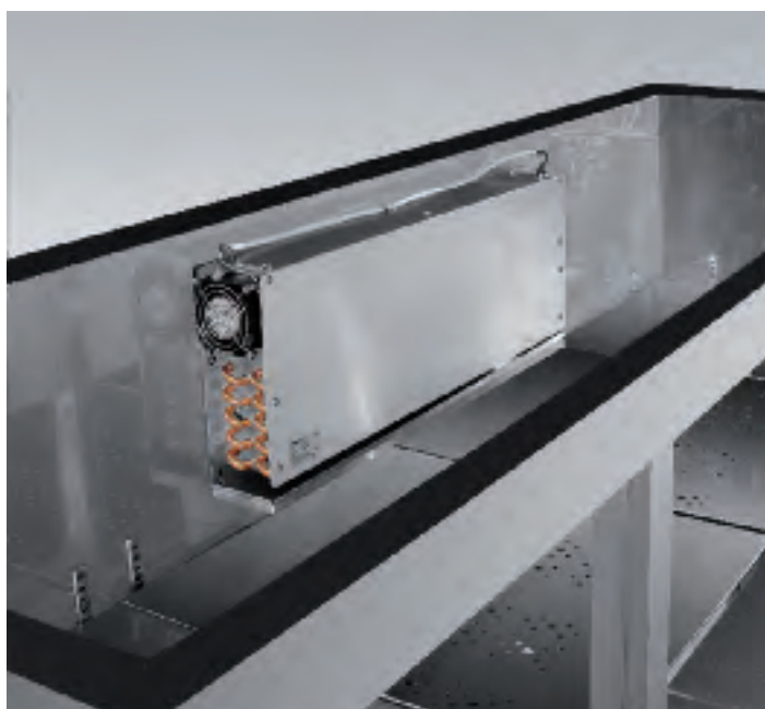
Esempi di installazione di evaporatore ventilato fissato a parete. Examples of installation of ventilated evaporator fixed to the wall.
