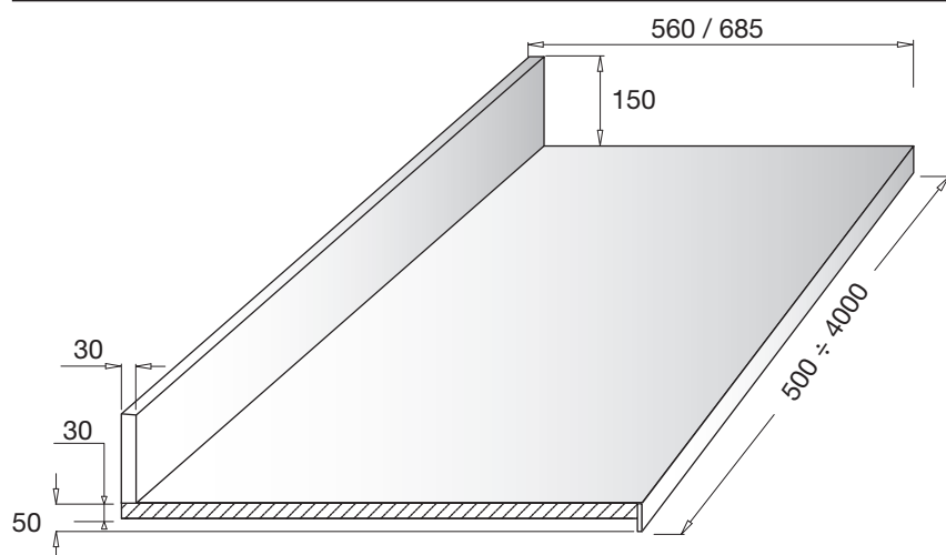
Piano con alzatina posteriore • Top with splashback
