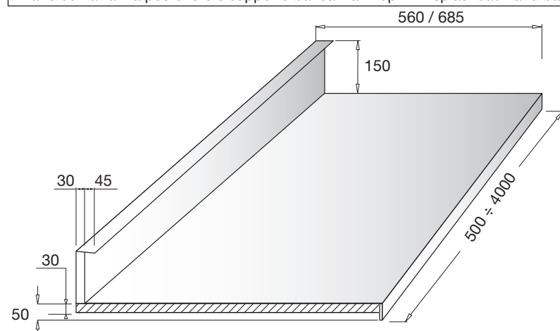
Piano con alzatina posteriore e supporto bancalina • Top with splashback and bar counter top holder
